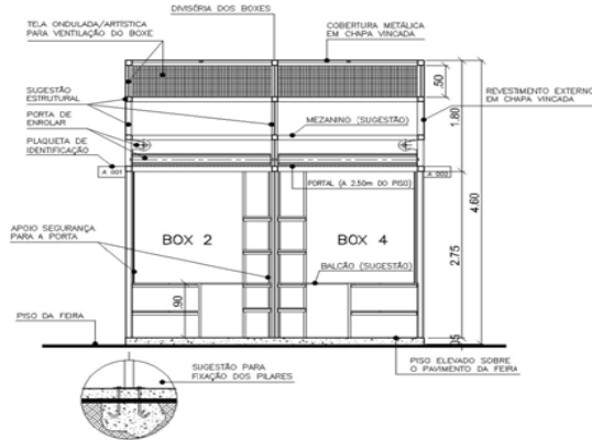
VII CORTE ESQUEMÁTICO MÓDULO C – BOXES 2x2m SEM ESCALA
