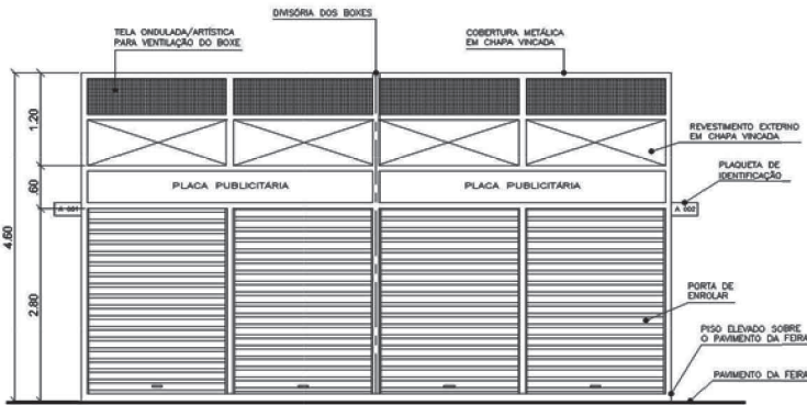
VIII EXEMPLO VISTA DOS BOXES SEM ESCALA
