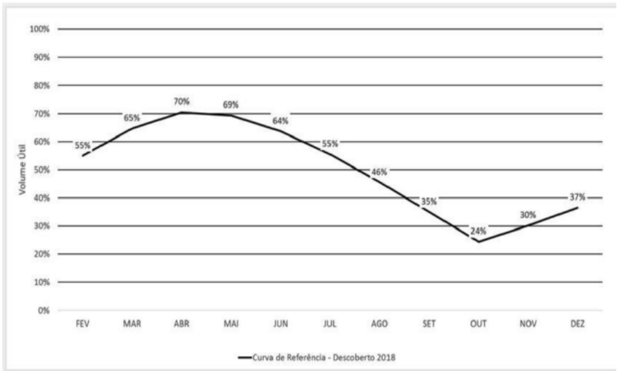
Figura 1 - Curva de referência do volume útil do reservatório do Descoberto.
