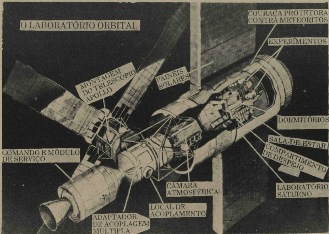
LABORATÓRIO ORBITAL DOS EUA - A concepção artística da foto apresenta as várias seções em que será dividido o futuro laboratório orbital que os Estados Unidos pretendem lançar ao espaço em 1972. O laboratório, propriamente dito, ocupa o cilindro maior, contido no terceiro estágio de um foguete Saturno. A energia elétrica é obtida de painéis solares em forma de moinho (USIS)
