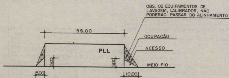
MEDIDAS MÁXIMAS PLL - Planta Baixa
