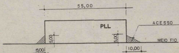
MEDIDAS MÁXIMAS PLL - Planta baixa
