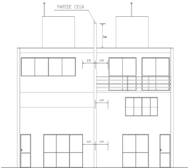
Figura 2 - Exemplo de projeção da parede cega
