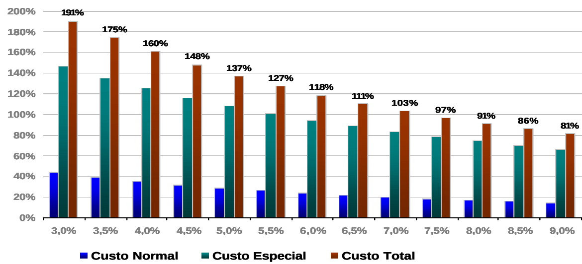
Variação dos Custos Normal, Especial e Total em relação à variação da taxa real anual de juros:
