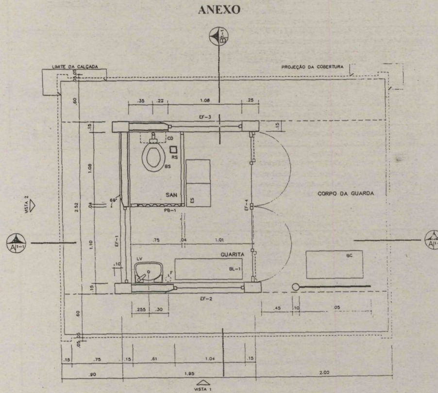
Planta Baixa Escala 1:20
