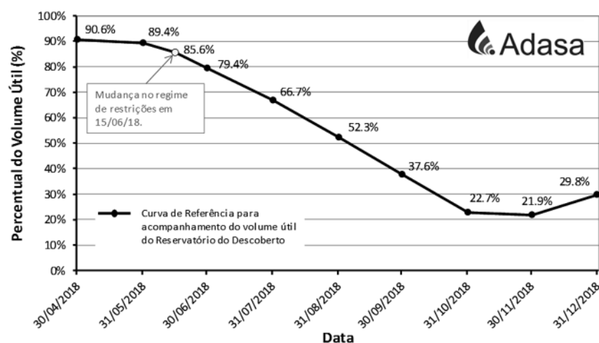
Figura 1 - Curva de referência para o acompanhamento do volume útil do Reservatório do Descoberto no período de maio a dezembro de 2018.
