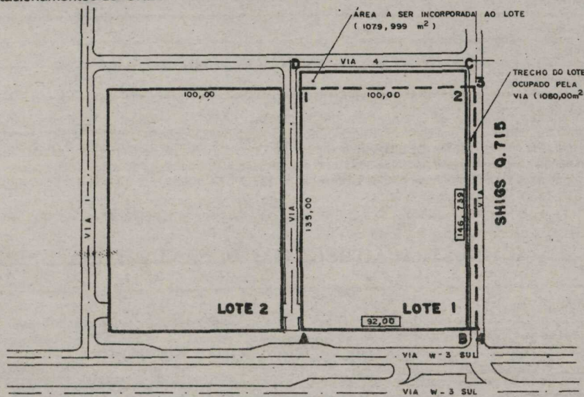
CROQUI 1 ESC.1:2000
