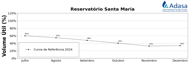
Figura 2 – Curva de referência para o acompanhamento do volume útil do reservatório do Santa Maria no período de julho a dezembro de 2024.
