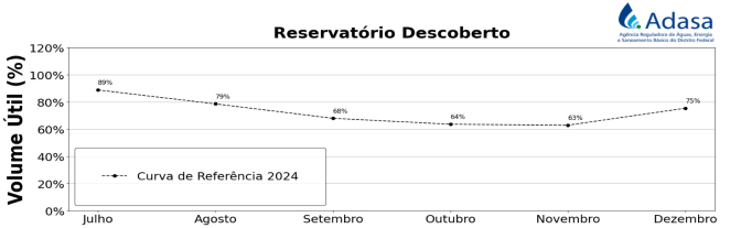
Figura 1 – Curva de referência para o acompanhamento do volume útil do reservatório do Descoberto no período de julho a dezembro de 2024.
