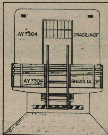
VISÃO DA ESCADA E PARTE ANTERIOR DA CASINHA
