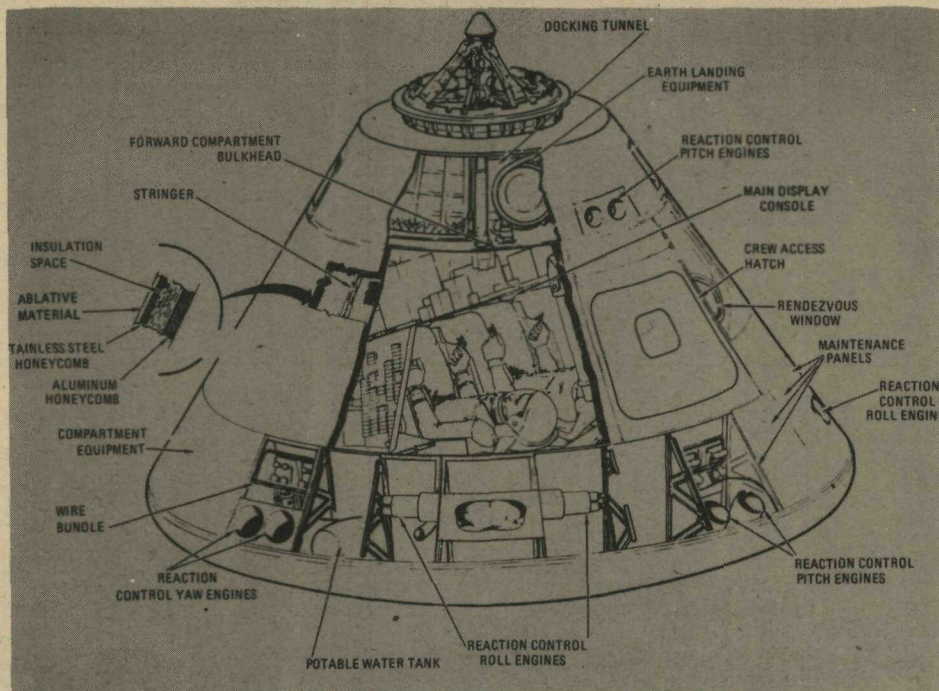
A APOLLO-11 - No gráfico da foto a nave espacial Apollo-11 é vista com todo o seu complexo instrumental indicado, vendo-se ainda a posição em que viajarão os três astronautas norte-americanos, quando do lançamento do gigantesco foguete Saturno V, em cuja ogiva estará a Apollo-11
