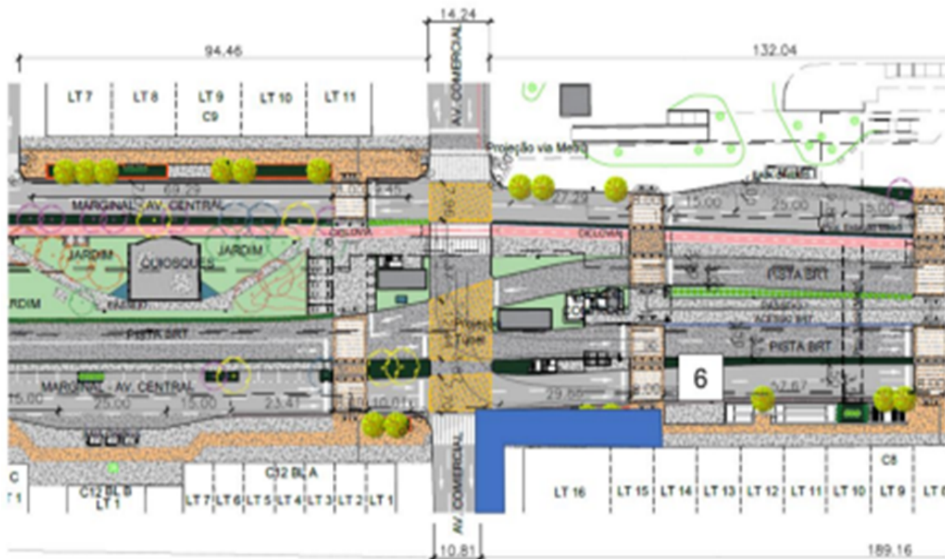
Figura 5: Ajuste de projeto para criação de passeio compartilhado que permitirá a interligação de ciclovias previstas na Comercial Sul e Av. Boulevard.
