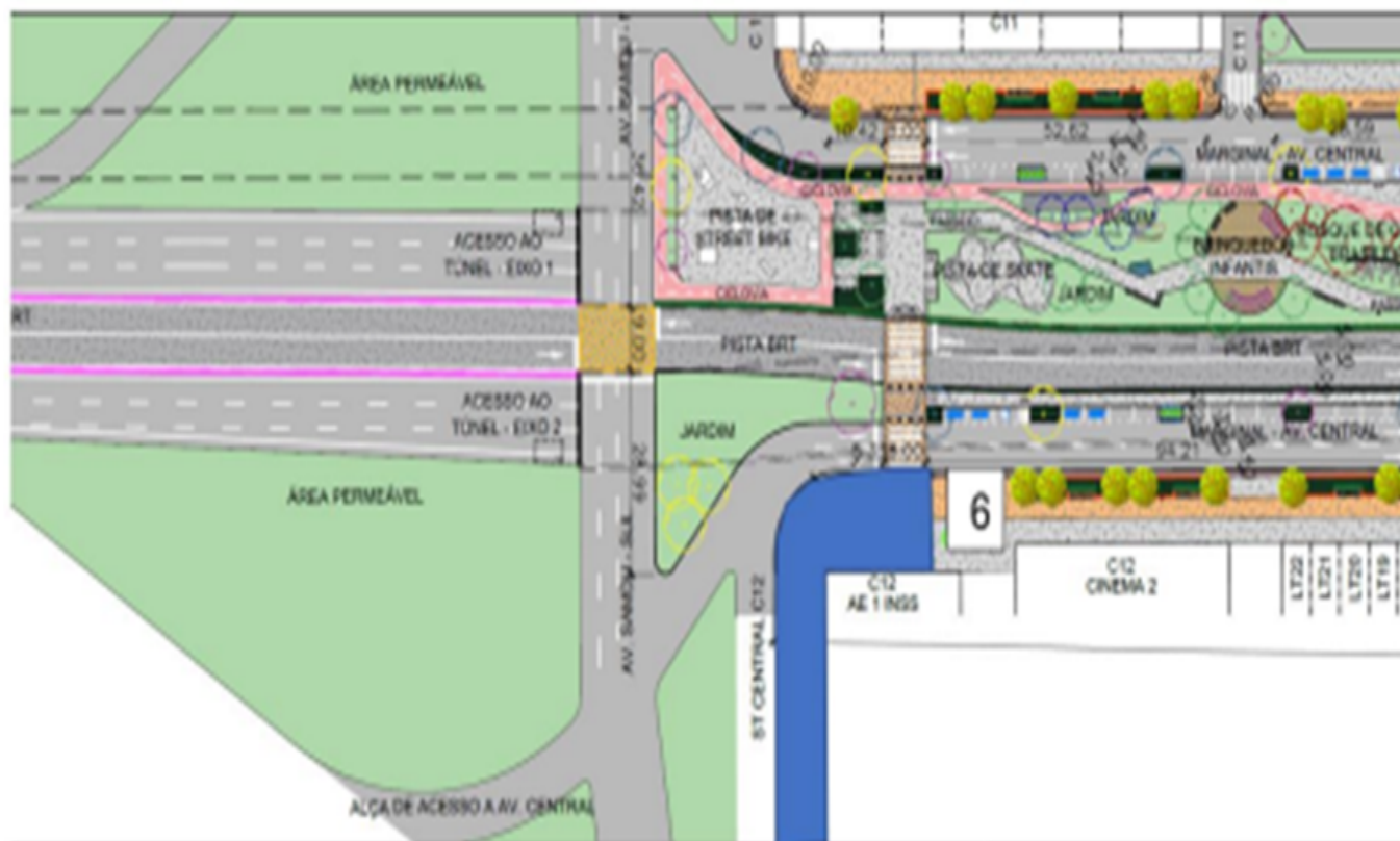
Figura 6: Ajuste de projeto para criação de passeio compartilhado que permitirá a interligação de ciclovias previstas na SAMDU e Av. Boulevard.
