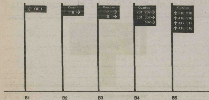
Suportes B Esc. 1:25
