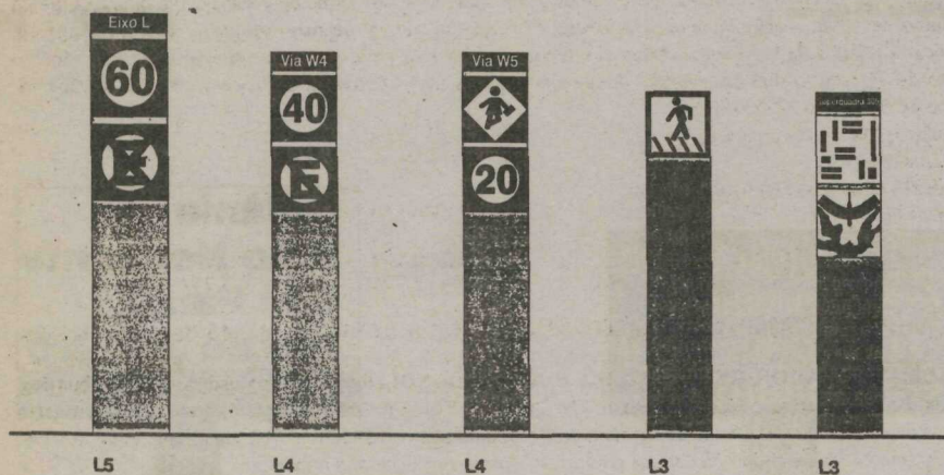
Suportes L - Regulamentação/Advertência/Serviço/Mapa e Diagrama de Quadra Esc. 1:25
