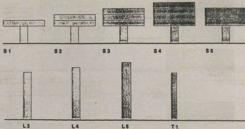
Suportes tipo: S, L e T Esc. 1:50
