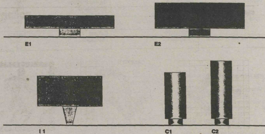
Suportes tipo: E, I e C Esc. 1:50
